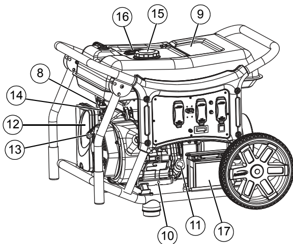
Figura 2-1. Características y controles
