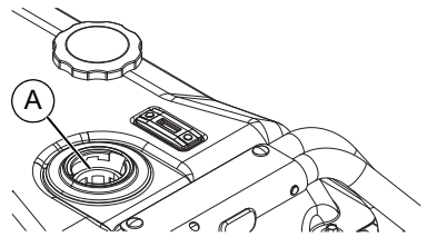
Figura 2-10. Cómo añadir el combustible recomendado
