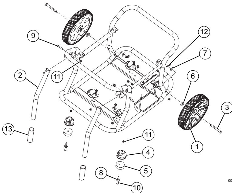
Figura 2-7. Armado de rueda, bastidor y pie
