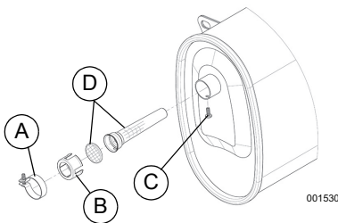
Figura 4-6. Tamiz del supresor de chispas
