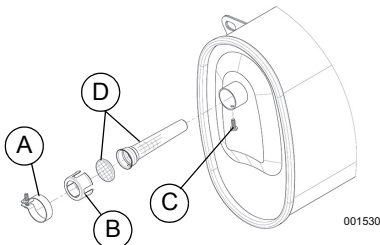
Figure 4-6. Écran pare-étincelles
