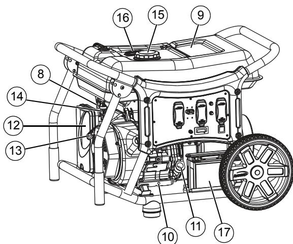
Figure 2-1. Caractéristiques et commandes
